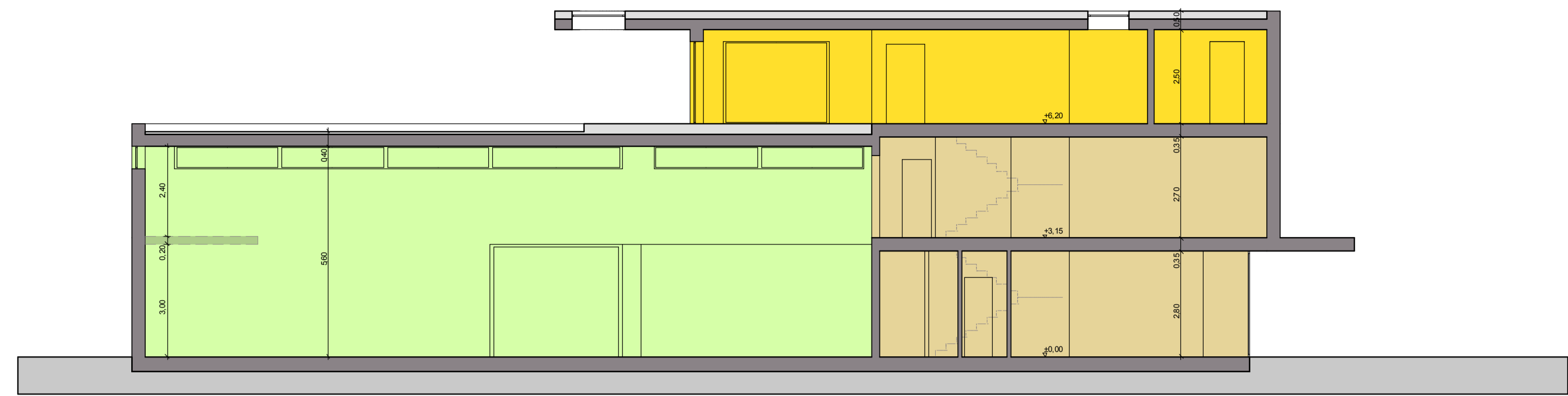
SCHNITT A-A 1:100
