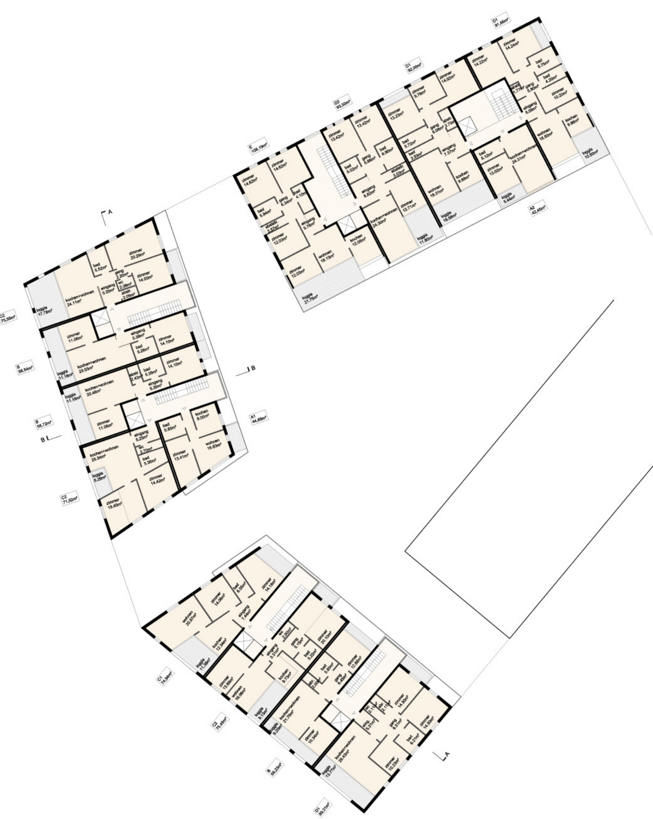
regelgeschoss (1. + 2. obergeschoss)
