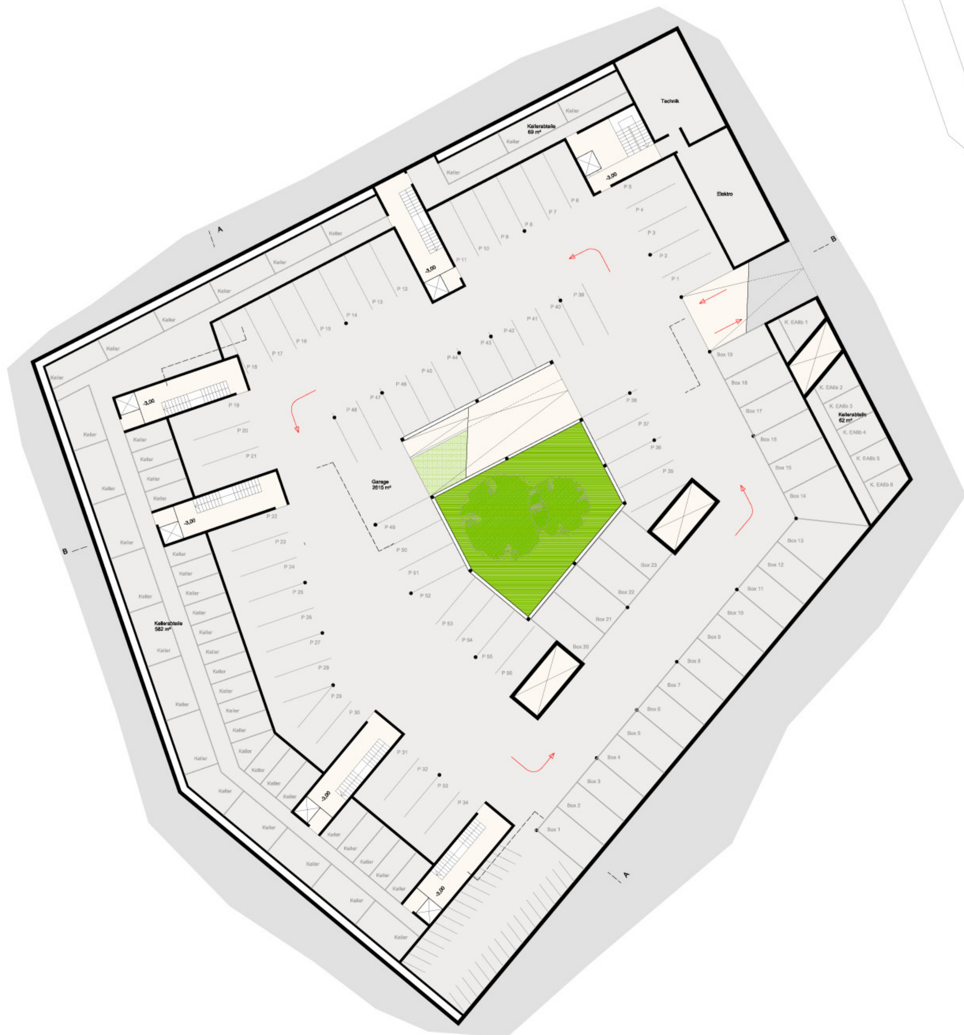
kellergeschoss 1
