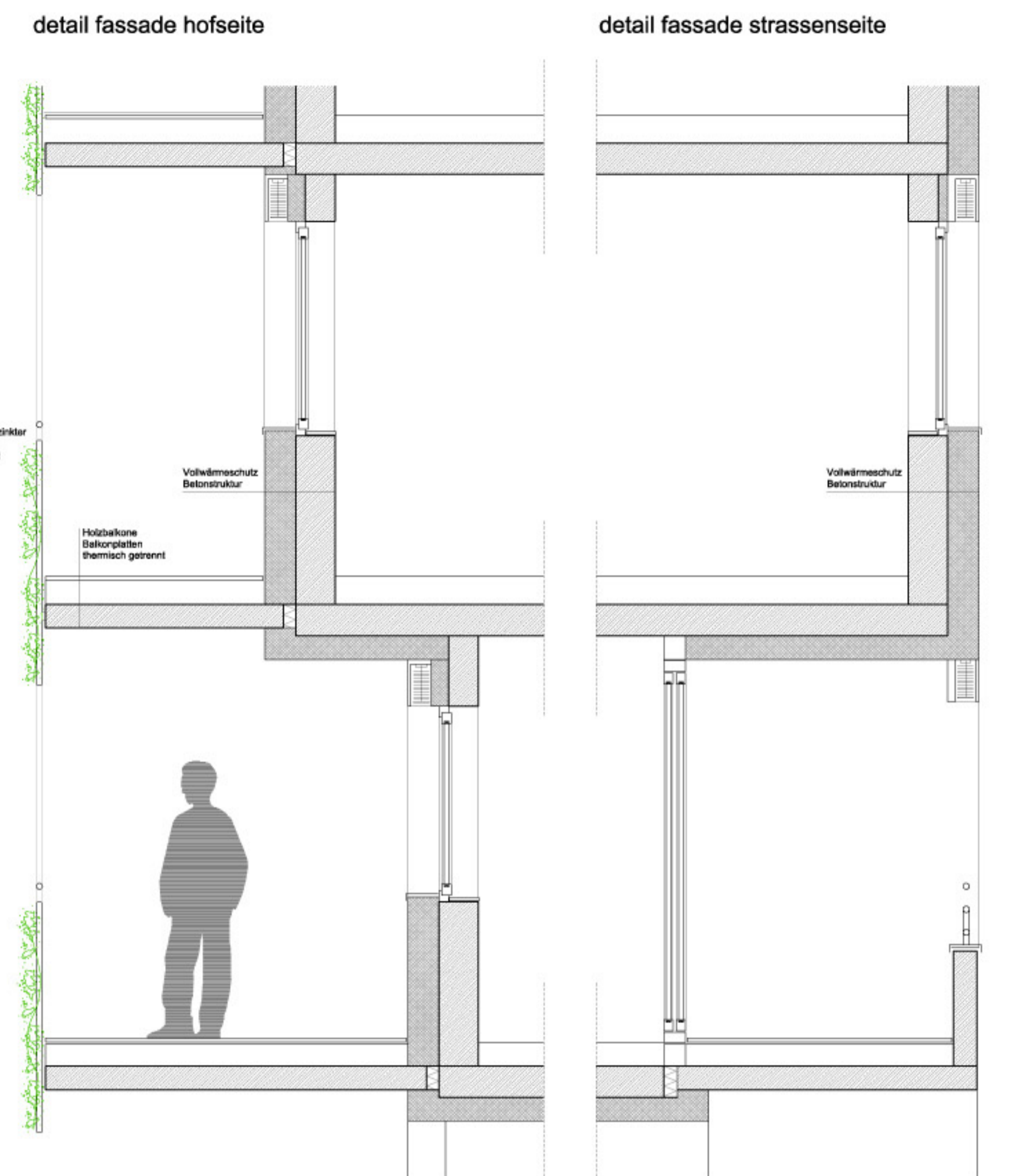
fassadenschnitt 1.25
