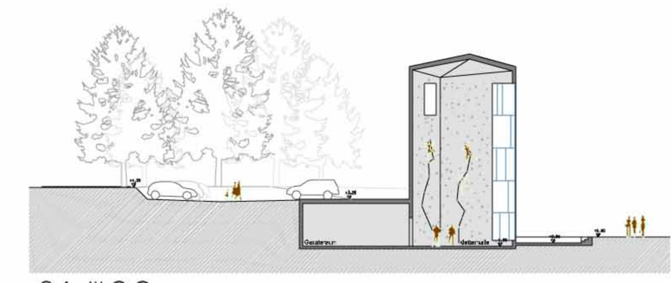
Schnitt G-G
