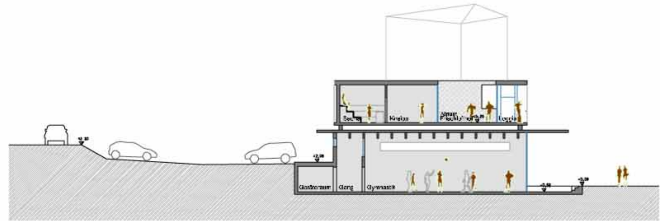
Schnitt D-D
