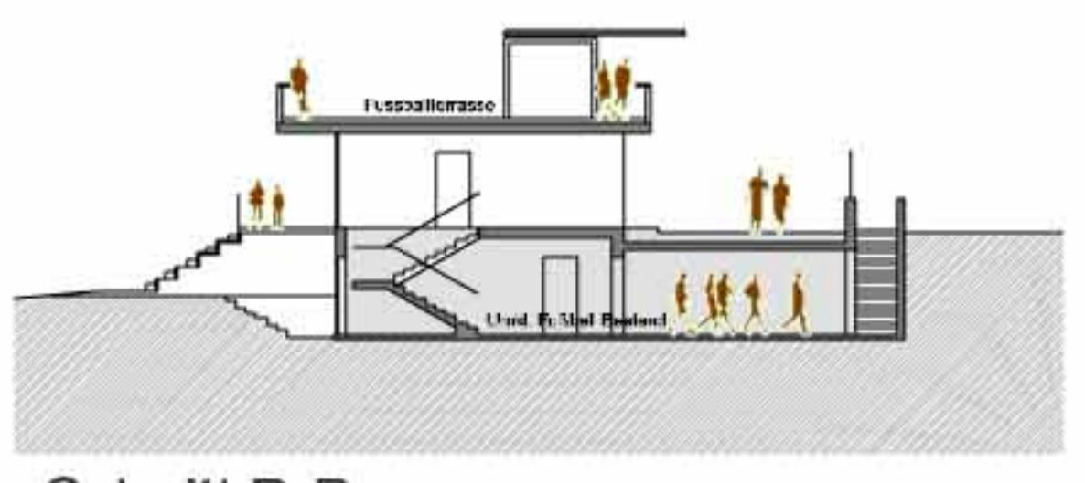
Schnitt B-B
