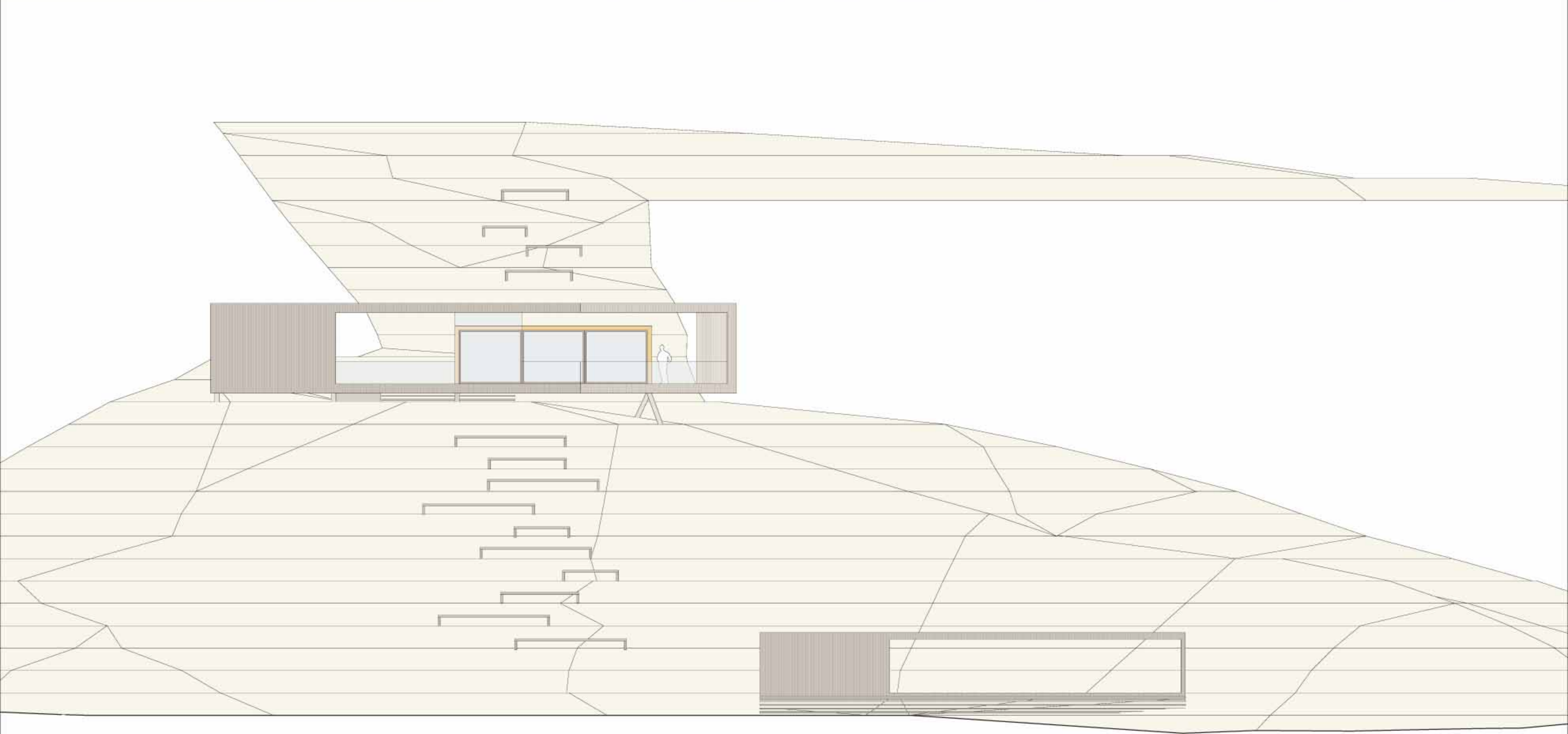
Ansicht West 1/100
