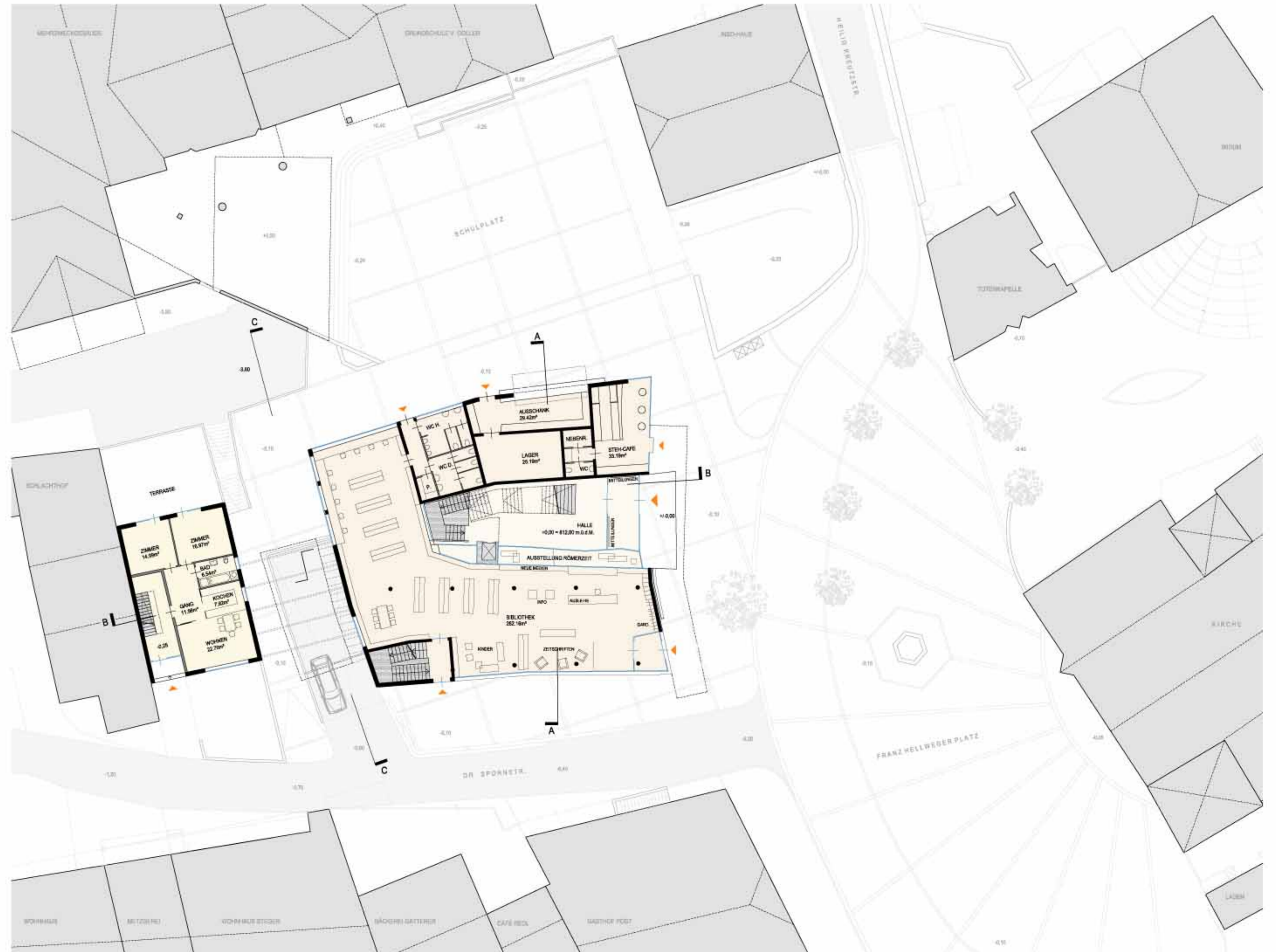
ERDGESCHOSS
