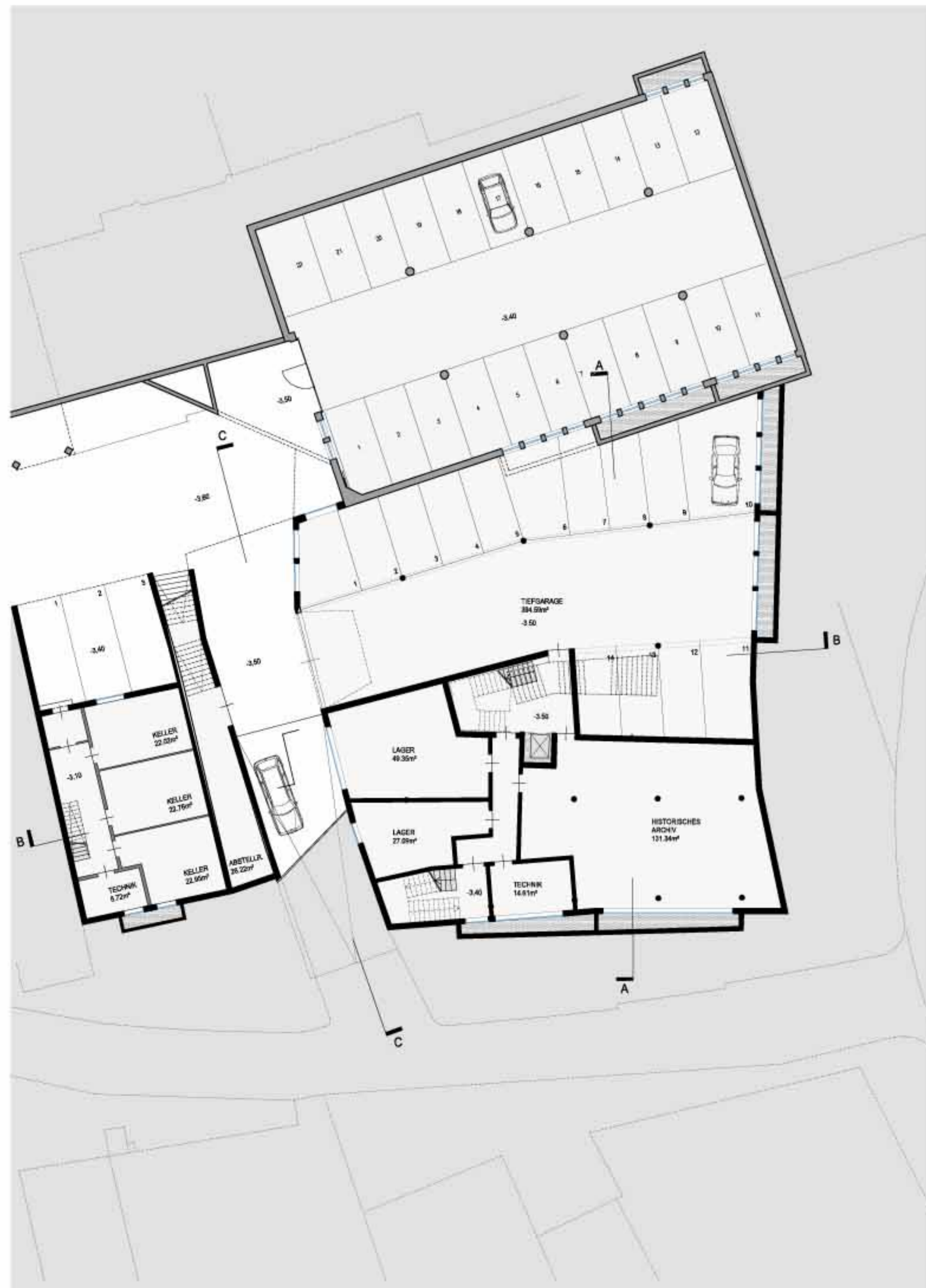
1. UNTERGESCHOSS
