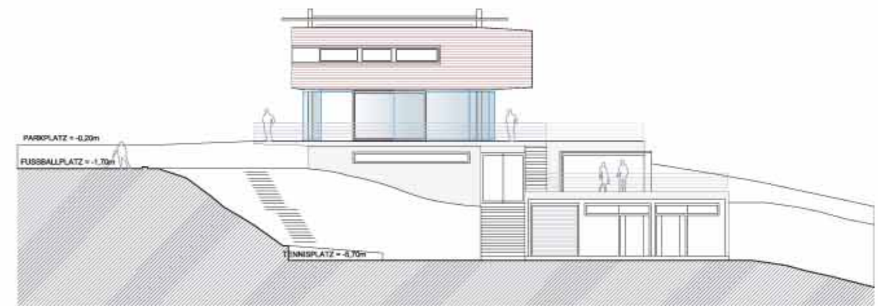
ANSICHT WEST
