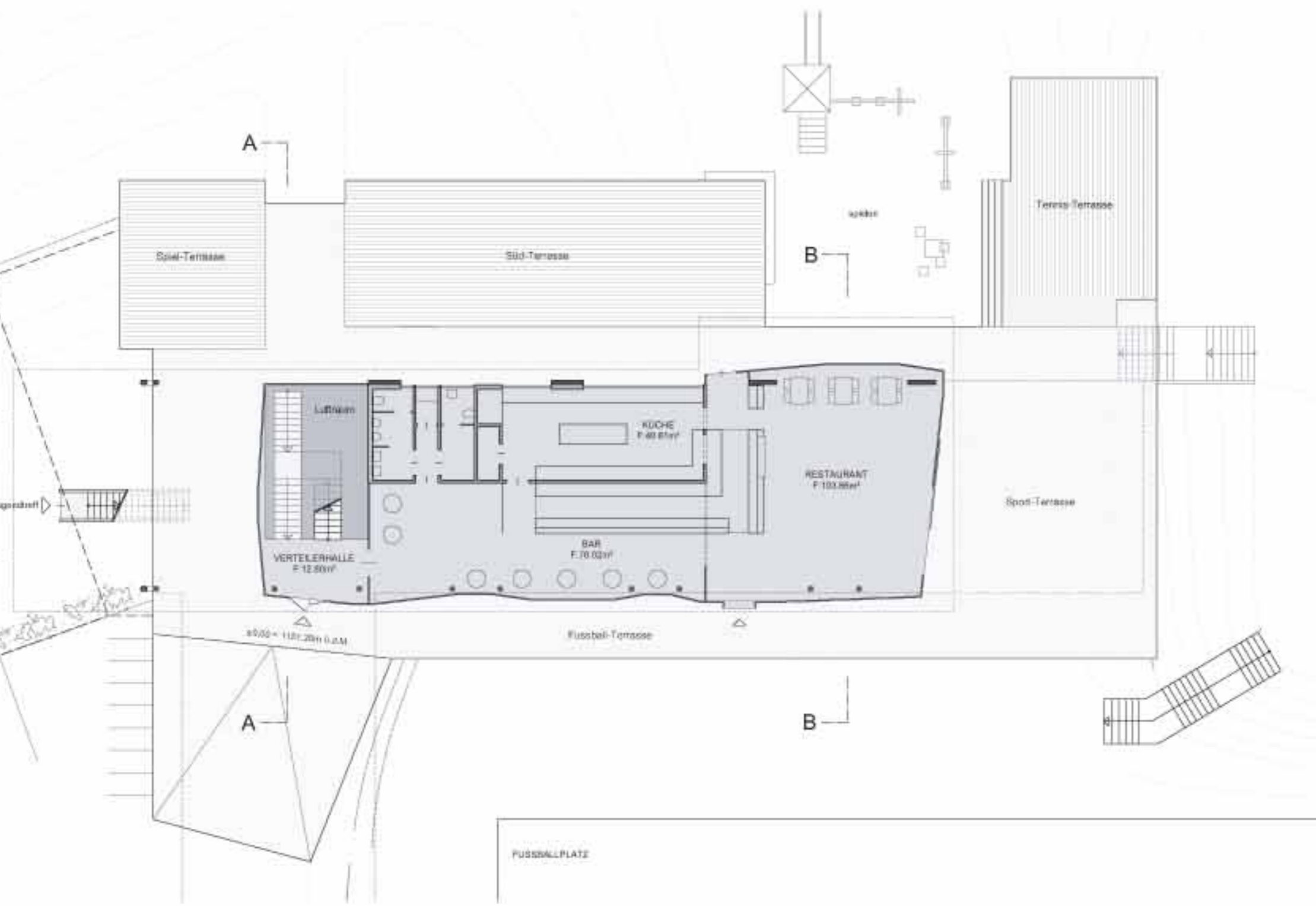
GRUNDRISS EBENE 0
