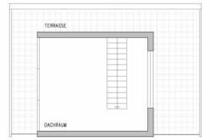
GRUNDRISS OG 2
