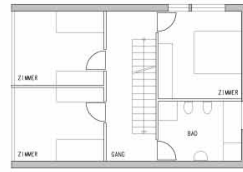
GRUNDRISS OG 1
