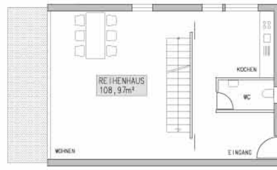
GRUNDRISS EG TYP 1
