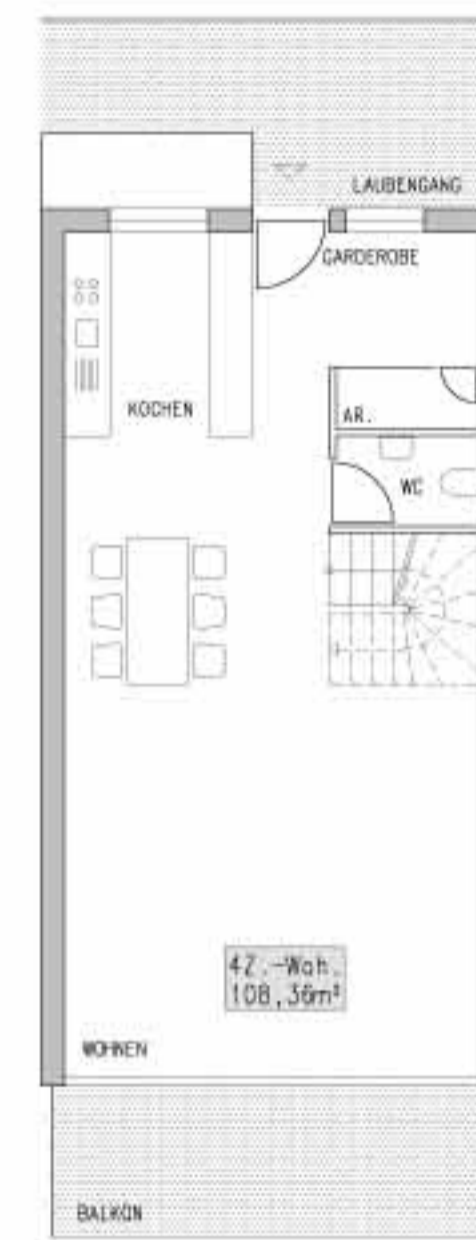
4-ZIMMER-WOHNUNG – ZWEIFGESCHOSSIG TYP 3
