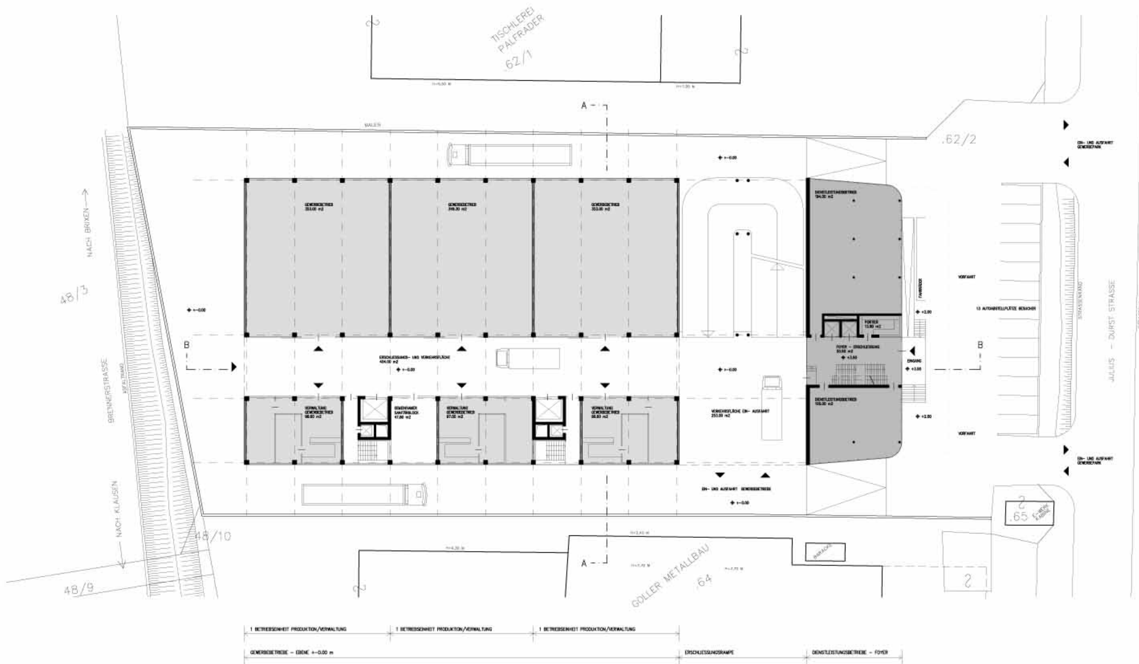
GEWERBEETRIEBE EBENE +/-0.00 m – DIENSTLEISTUNGSBETRIEBE EBENE +3.50 m M. 1 : 200
